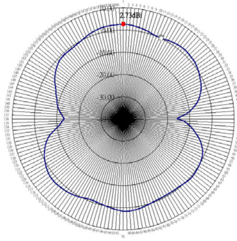
H-Plane
