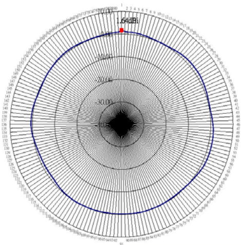
E-Plane
