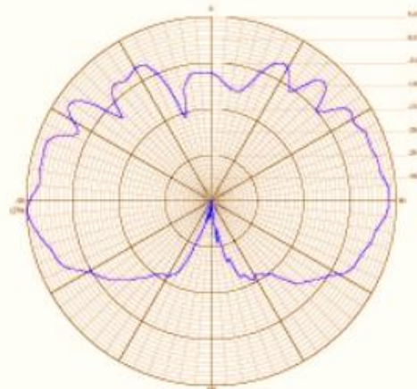
5750 MHz E-Plane
